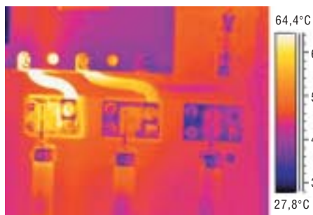
Anschluss mit hohem Übergangswiderstand
